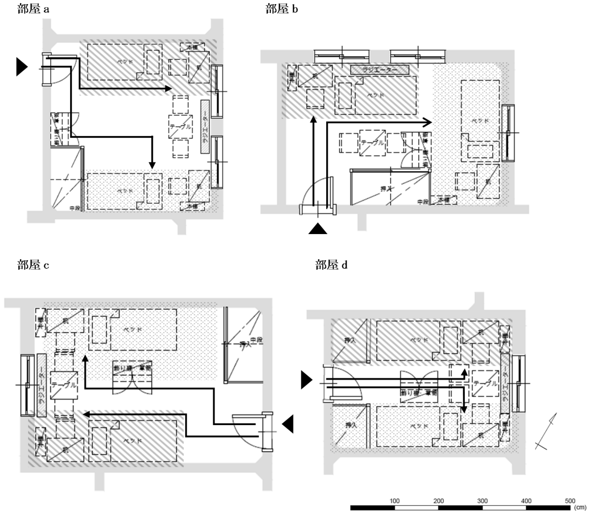
図3) 2人部屋平面図 a, b, c, d
