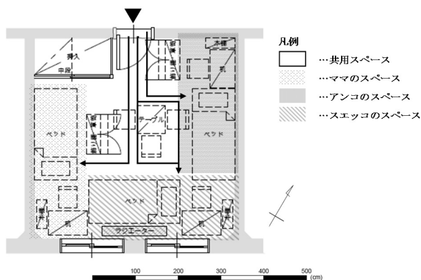
図2) 3人部屋平面図(ママは年長者、スエッコは年少者、アンコは中間の学年)
