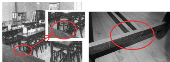
図10. 長机②の古写真比較（左：日本女子大学学寮100年研究会編（2007）p.53より加工、中：左を拡大したもの、右：長机②のトンボ貫）
